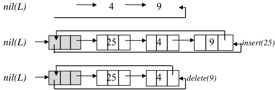
4 pav. Sąrašas, naudojantis signalinį žymenį.
