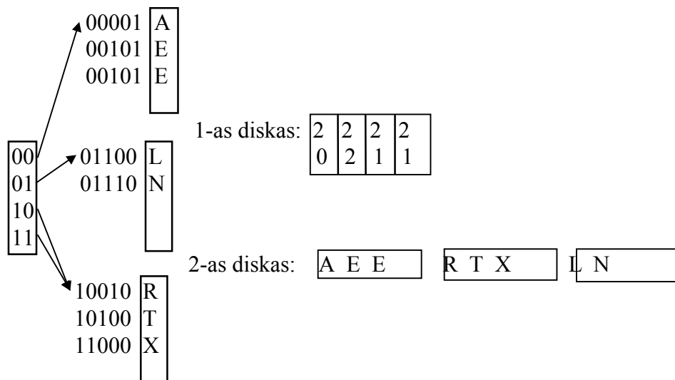
19 pav. Išplėstinio dėstymo struktūra diske.
