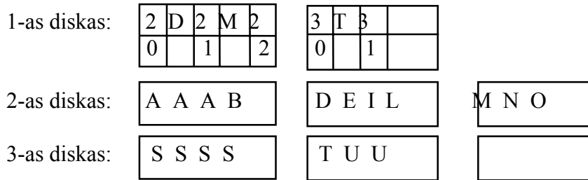
18 pav. Sakinio “SUBALANSUOTAS MEDIS” (žr. 11 pav.) B-medis diske.
