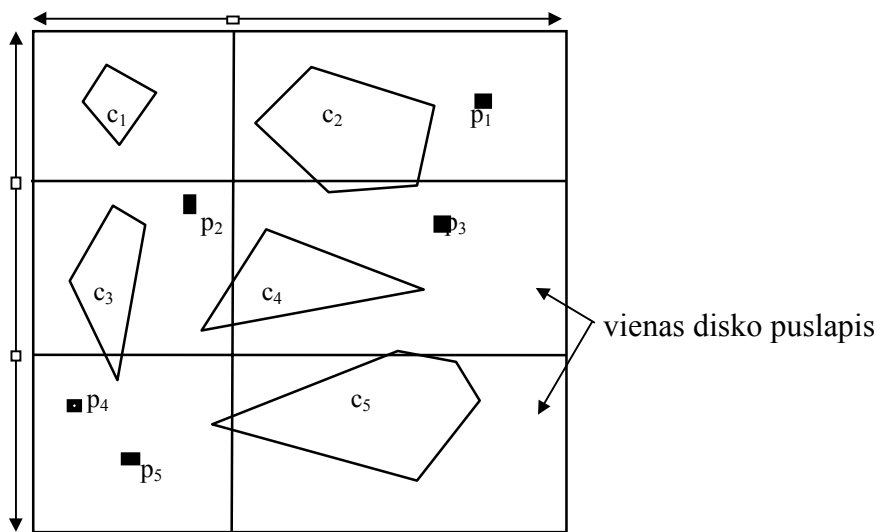
26 pav. Modelinio uždavinio grid file .
