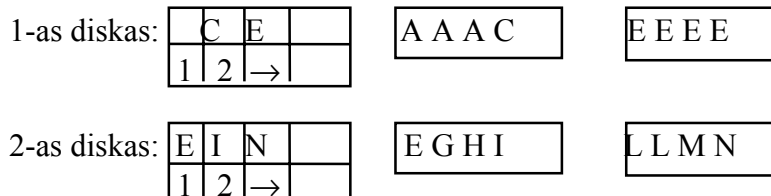
17 pav. Indeksinė-nuosekli struktūra diskuose.
