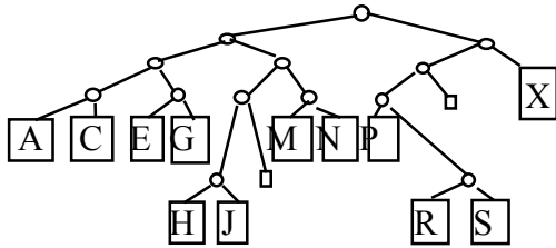
14 pav. Trie struktūra raidžių penkių bitų kodams.
