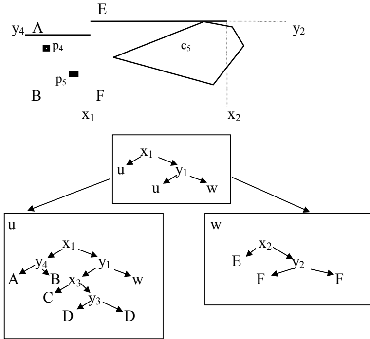
28 pav. Modelinio uždavinio hB-medis.
