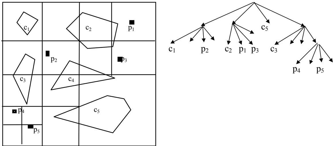
25 pav. Modelinio uždavinio sektorinis ketvirtainis medis.
