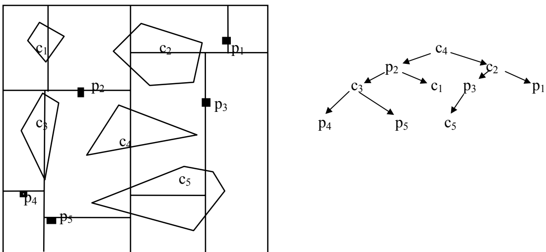
23 pav. Modelinio uždavinio k-d-medis.
