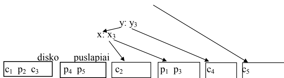
29 pav. Modelinio uždavinio LSD-medias.
